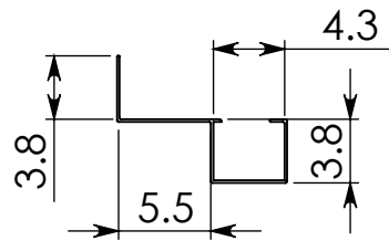
V frontal
